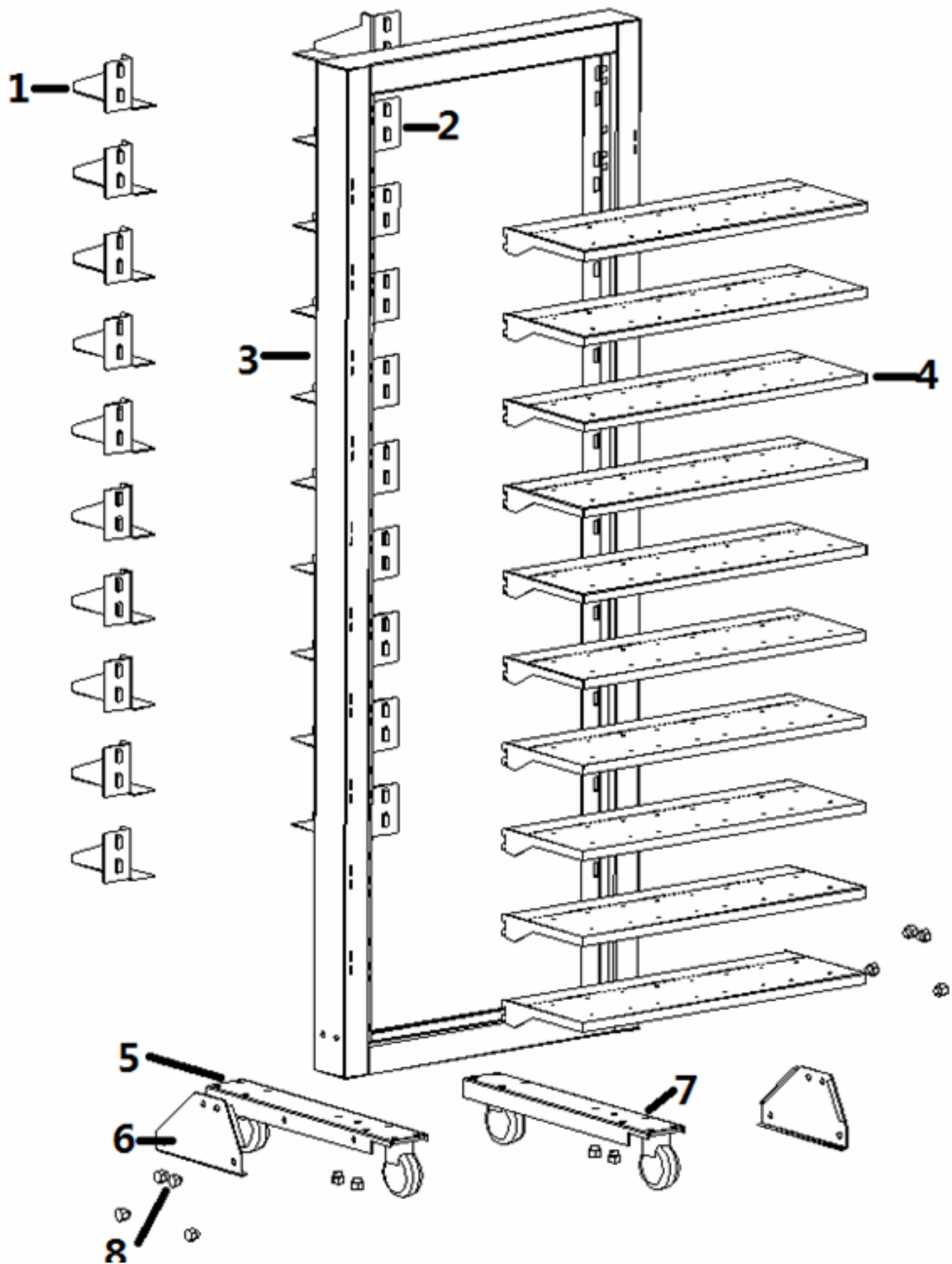
1— Left steel holder 2— Right steel holder 3— 10-story rack 4— Shelf 5— Left wheel 6— Rack fixer 7— Right wheel 8— M8*15 Screws
